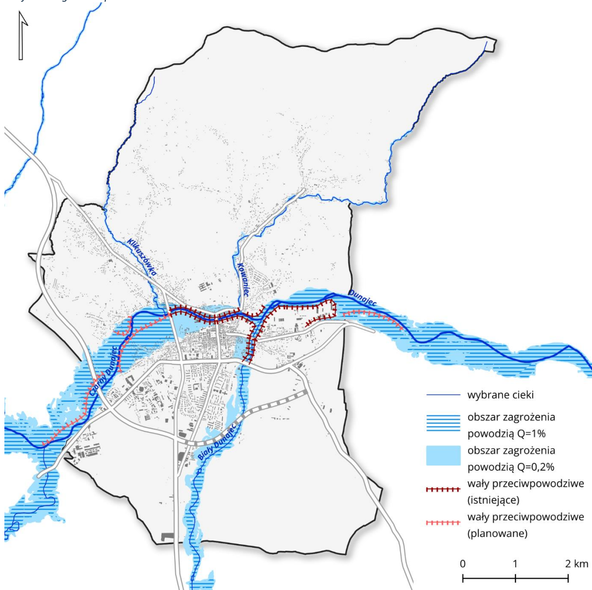
Grafika 8 Zagrożenie powodziowe na terenie miasta
